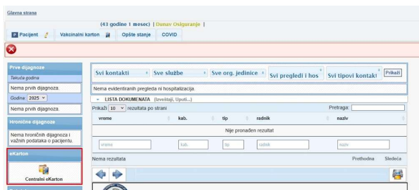
slika 1 – Pristup eKartonu
